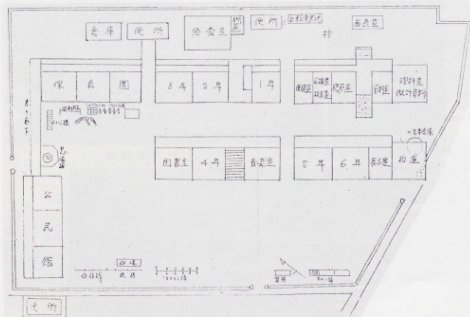
校地・校舎平面図 (更木教室)
