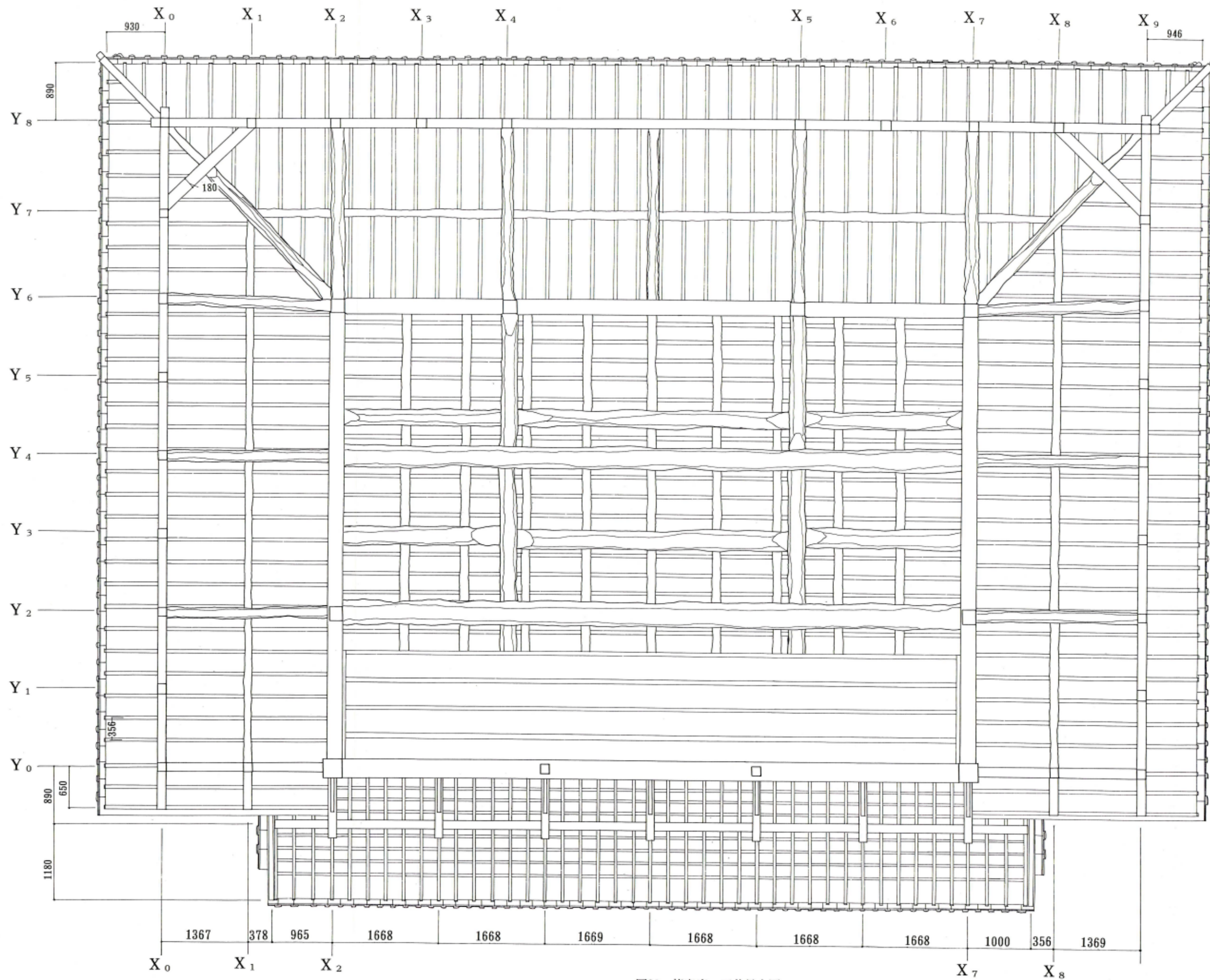
图23 皆楽座 天井見上図
