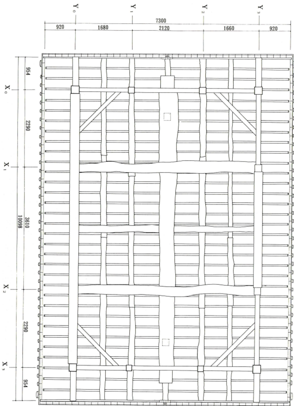
图5 赤坂神社拜殿 天井見上図
