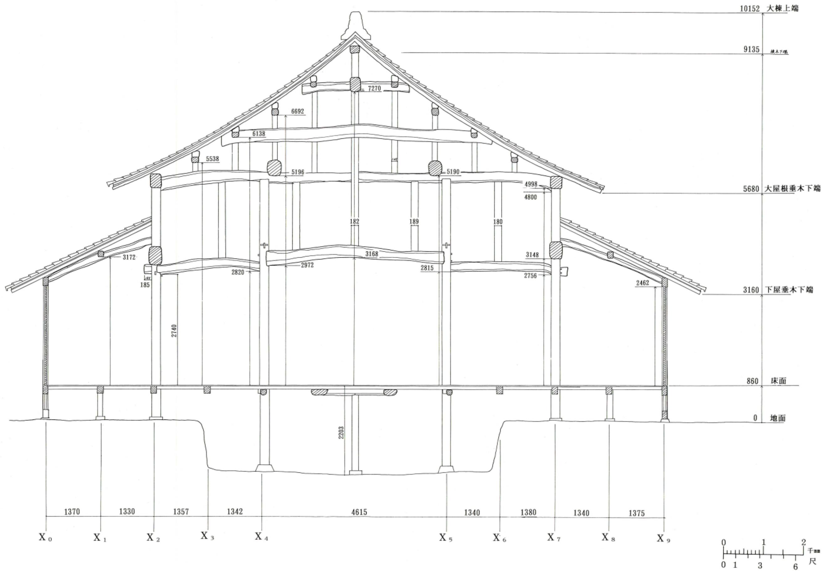
图25 皆楽座 梁行 (Y 5 ~ Y 6) 断面图
