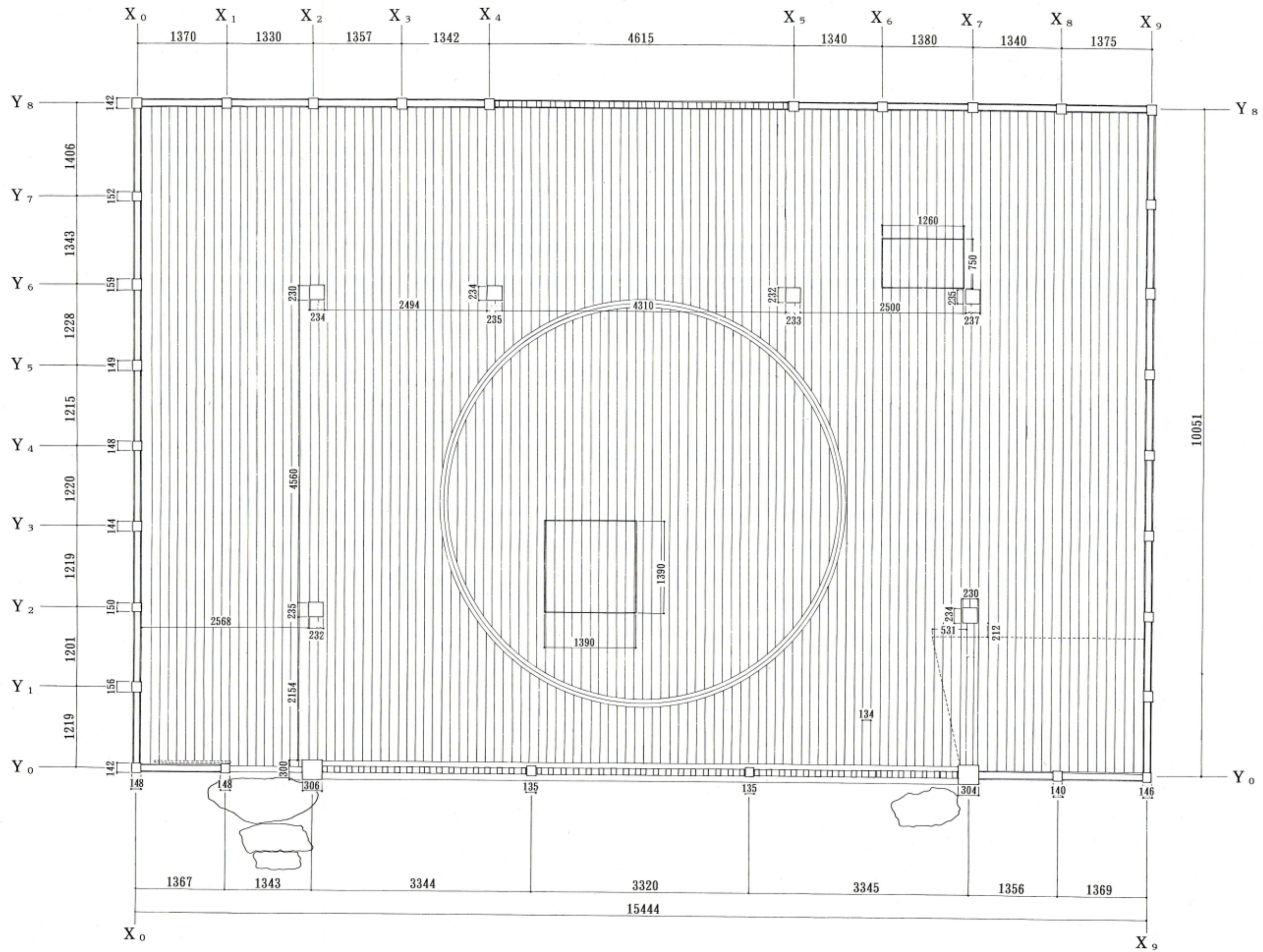
图18 皆乐座 一階平面图
