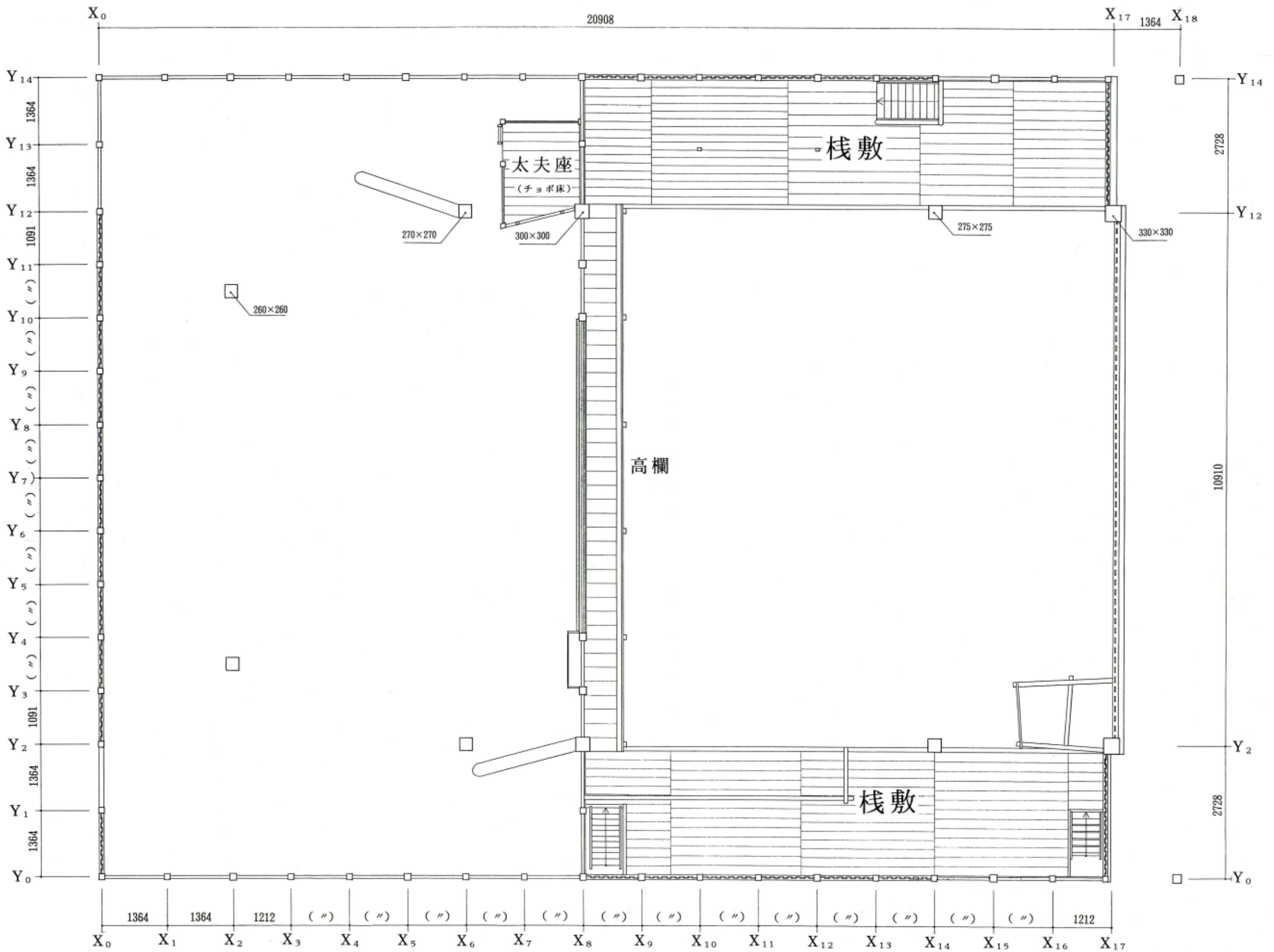
図29 村国座 二階平面図
