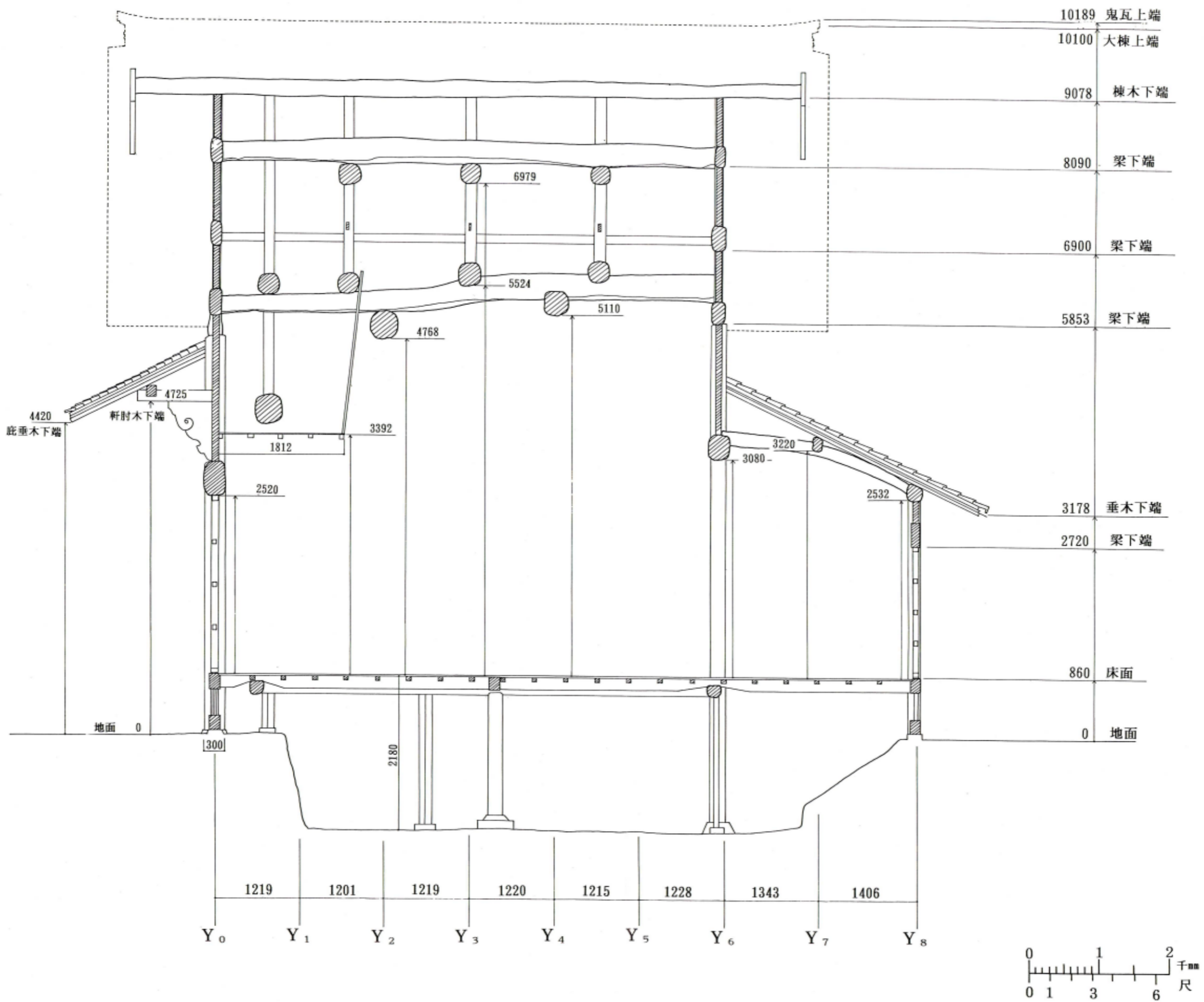
图26 皆楽座 桁行 (X 4 ~ X 5) 断面图
