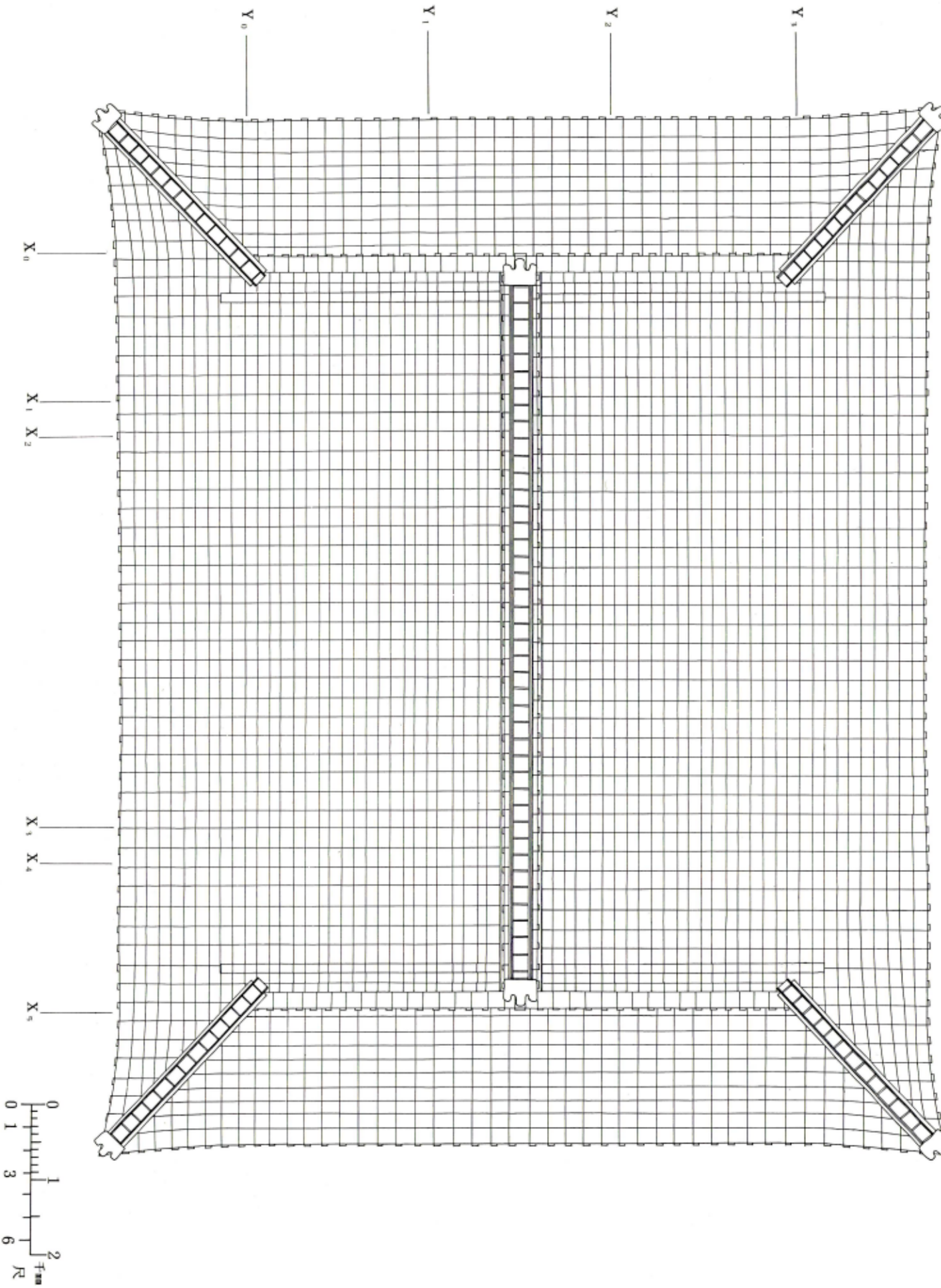
图15 二之宮神社舞台 屋根伏図
