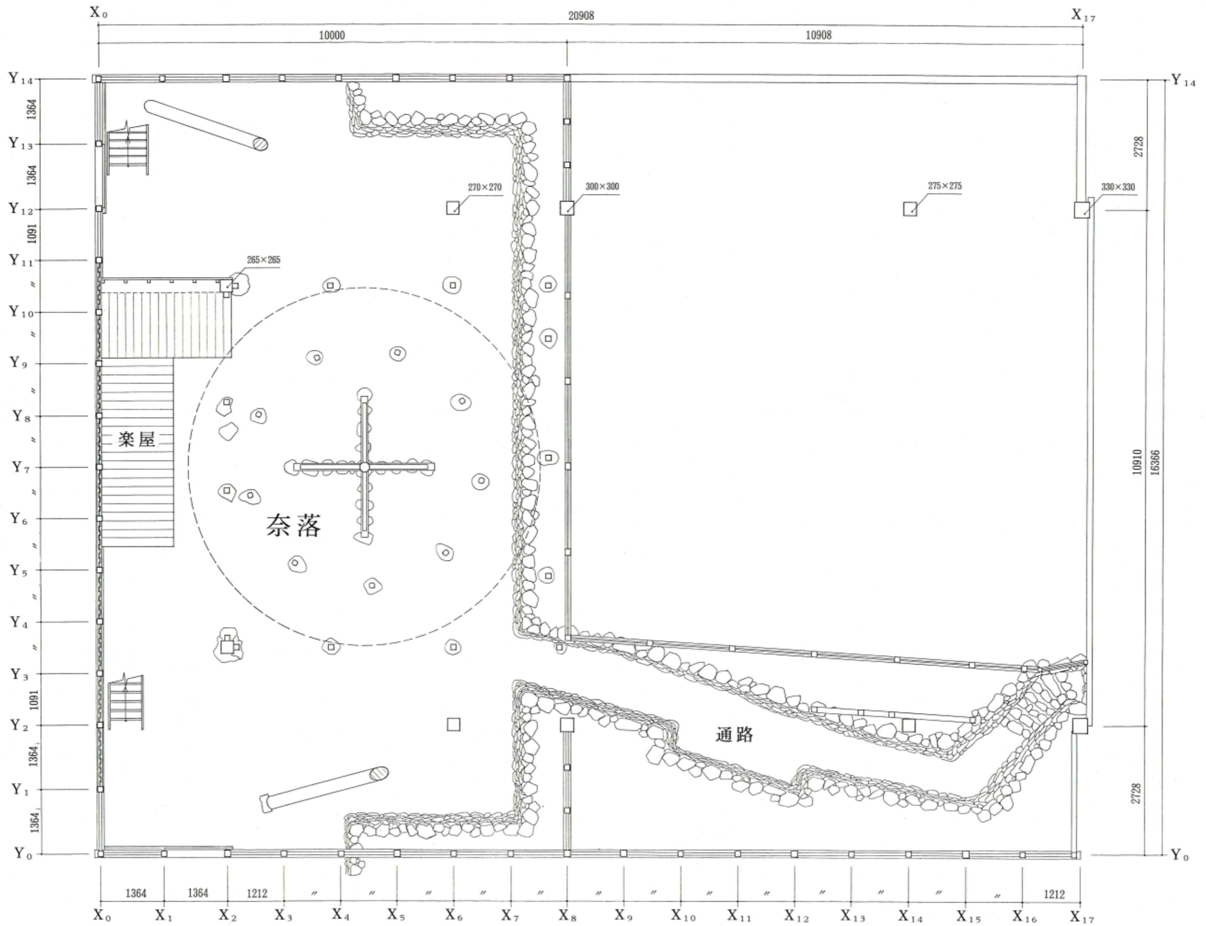
图30 村国座 地階平面图
