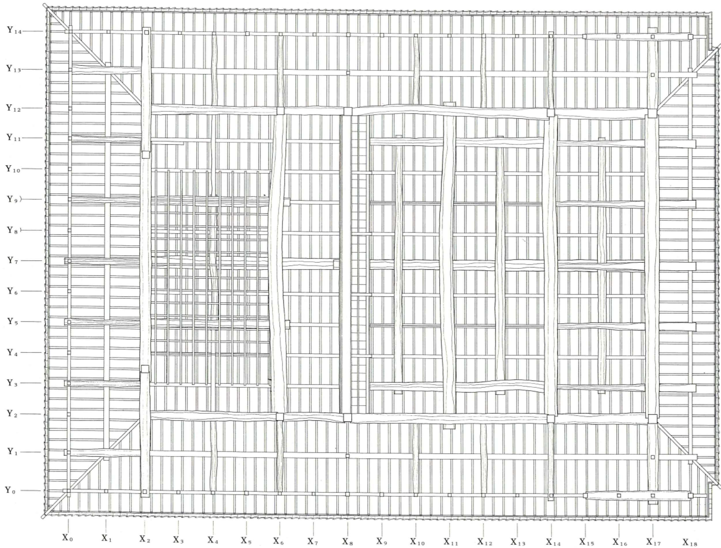
図35 村国座 天井見上図
