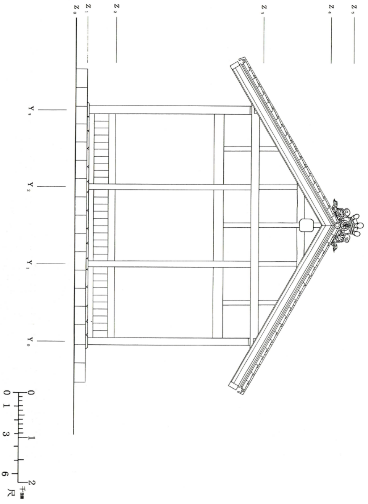
图50 春日神社拜殿 西立面图
